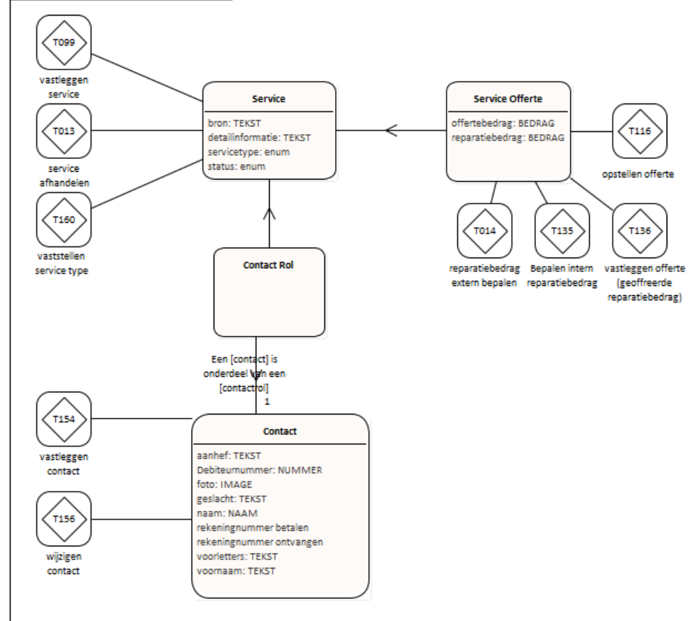
Object Fact Diagram OFD Afhandelen Service
